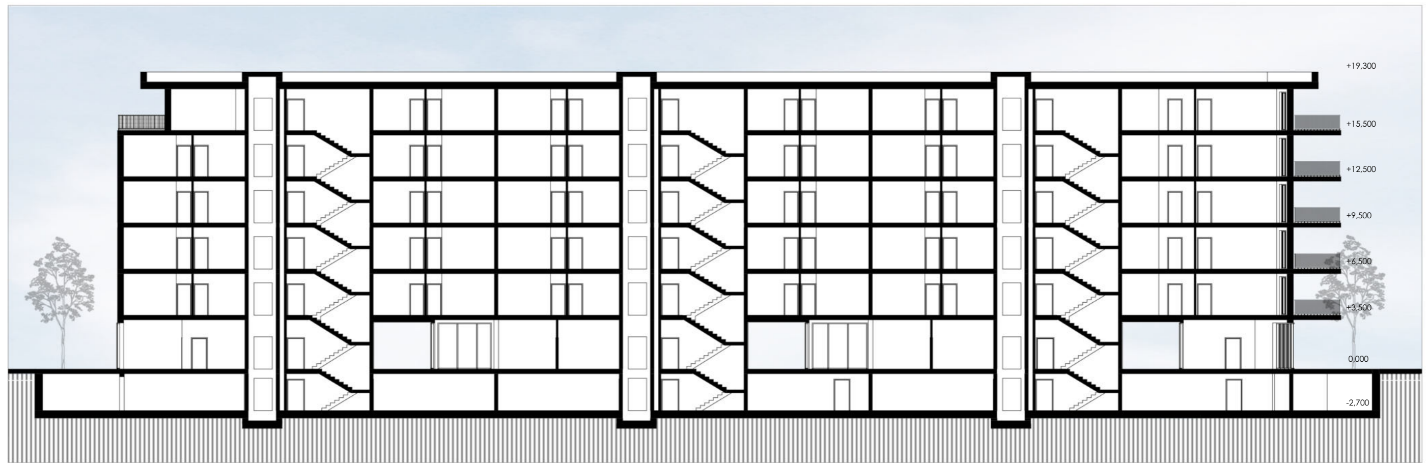
Rez A-A
