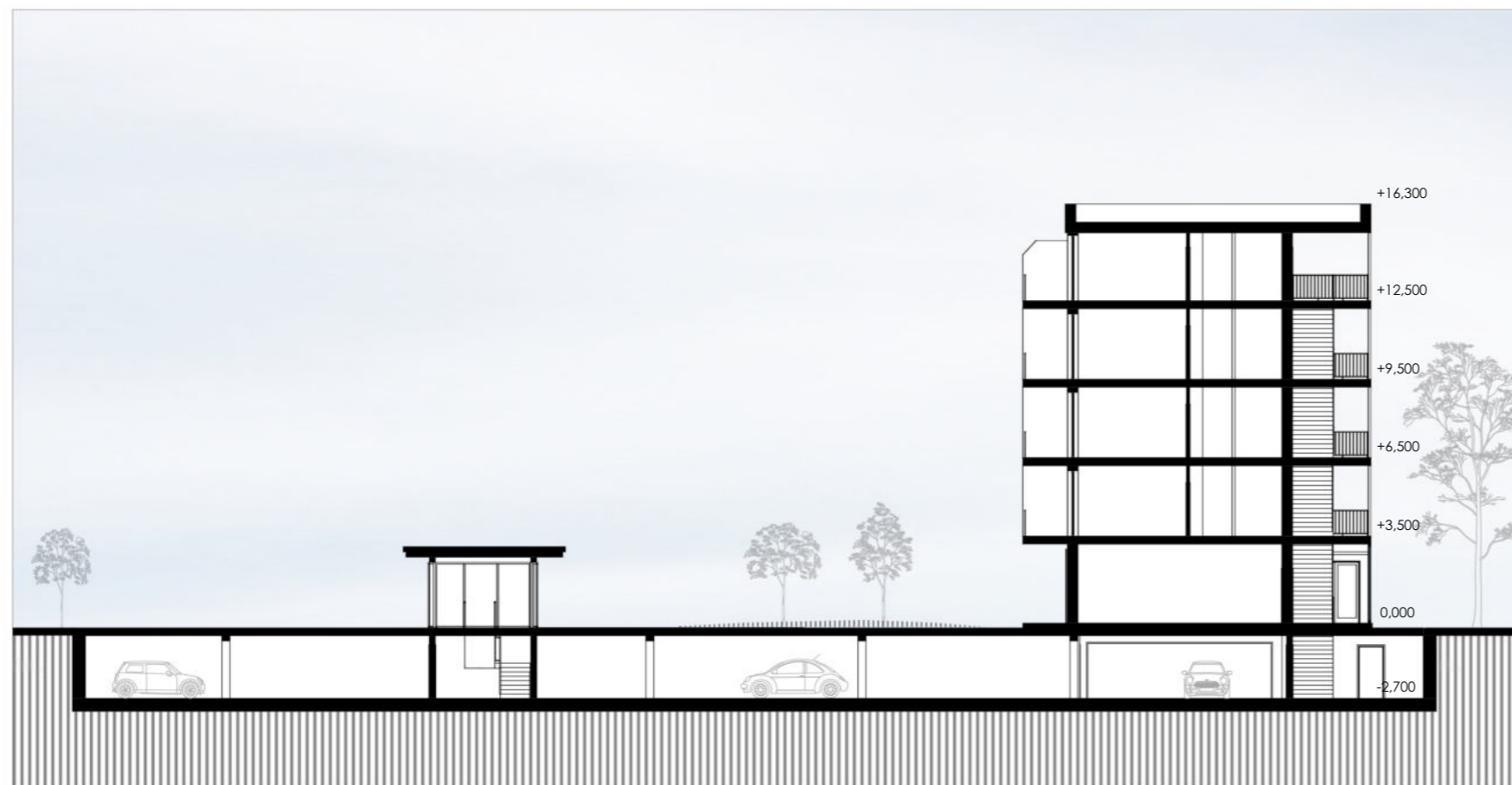
Rez D-D
