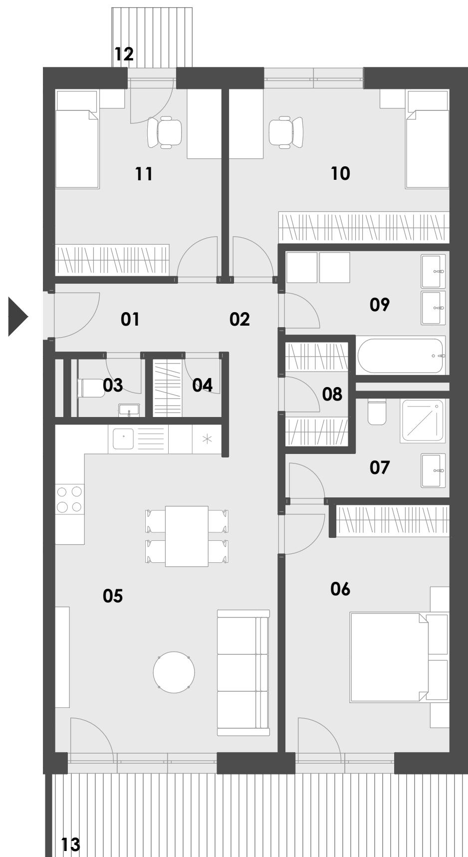
BYT 2.1 M 1:75
