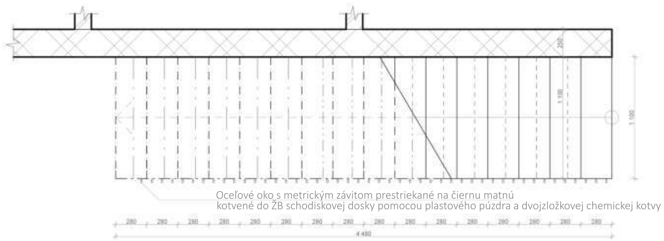
Pôdorys schodiska
